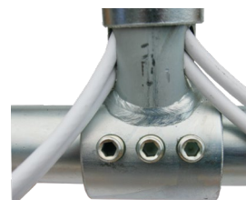
Sparrenbreite einstellbar
