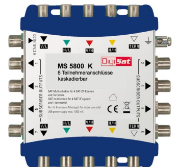
MS5800K | incl. Zubehör 9xDC-Endwiderstand, 9x18cm Verbindungskabel F-Stecker auf F-Stecker
